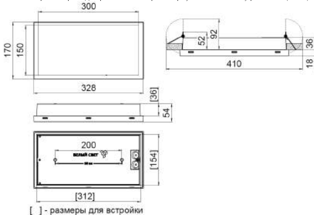
Рис. №2 Габаритный чертёж. Для крепления в гипсокартон потребуется комплект аксессуаров BS-КА-3 (a14565).
